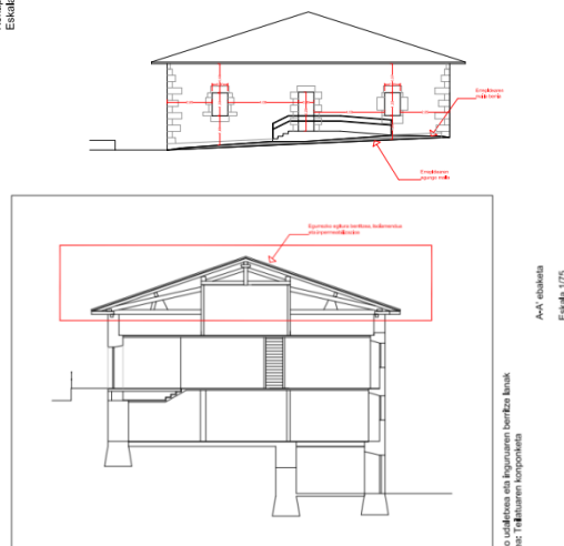
Eskaila: Eskala: 1/100
